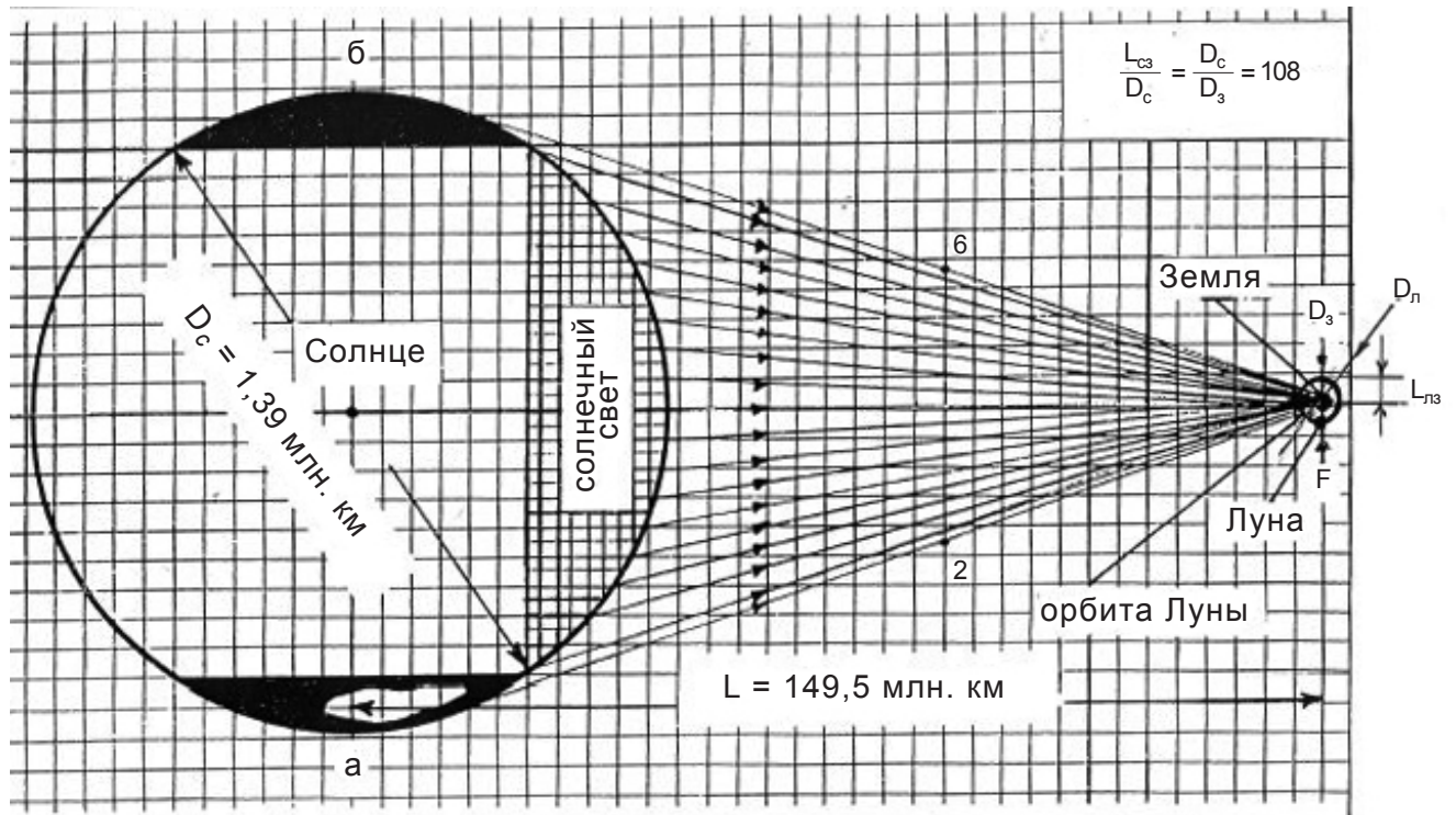
Рис. 1. Оптическая схема системы «Солнце - Луна - Земля». Открытие оптической схемы системы «Солнце - Луна - Земля» привело к определению оптического критерия «землеподобности» планет во Вселенной [3].
